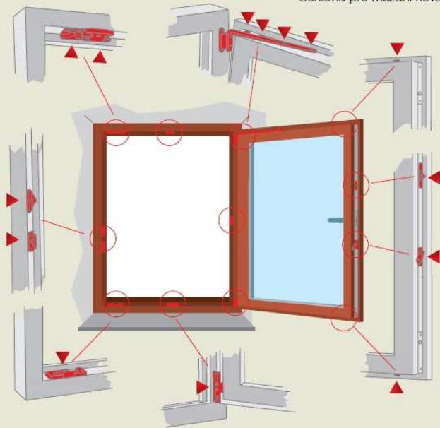
Schéma pro mazání kování
