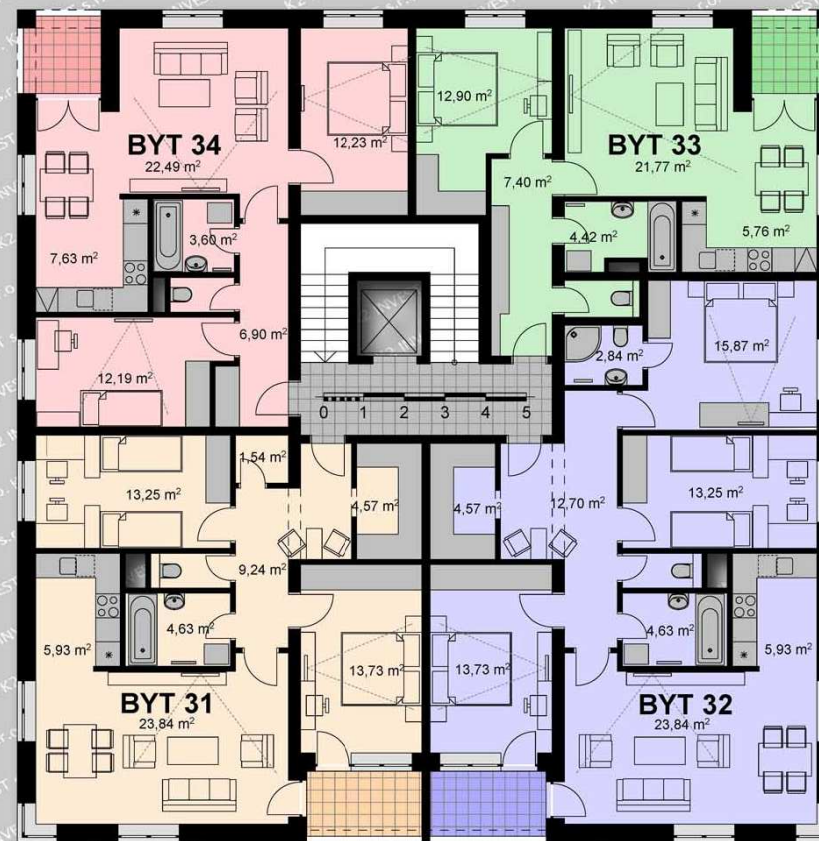
PŮDORYS 3.NP
