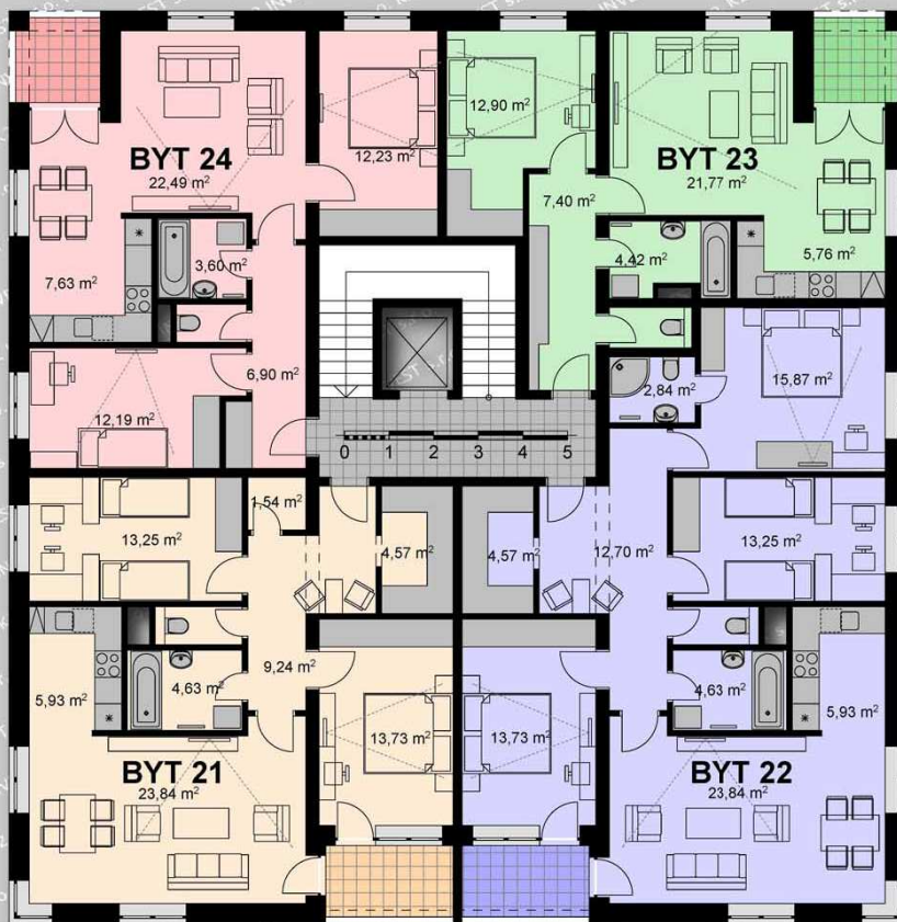
PŮDORYS 2.NP
